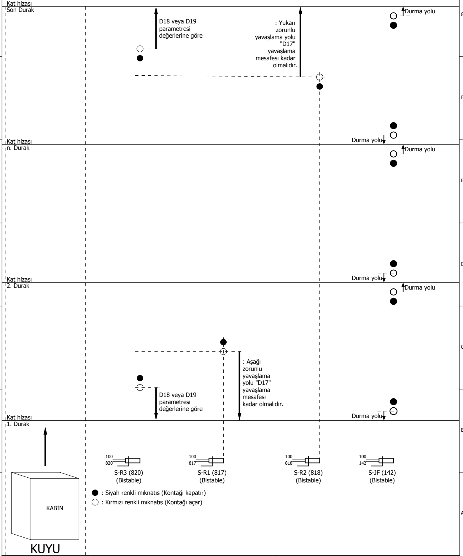
MIKNATIS DİZİLİM ŞEMASI
