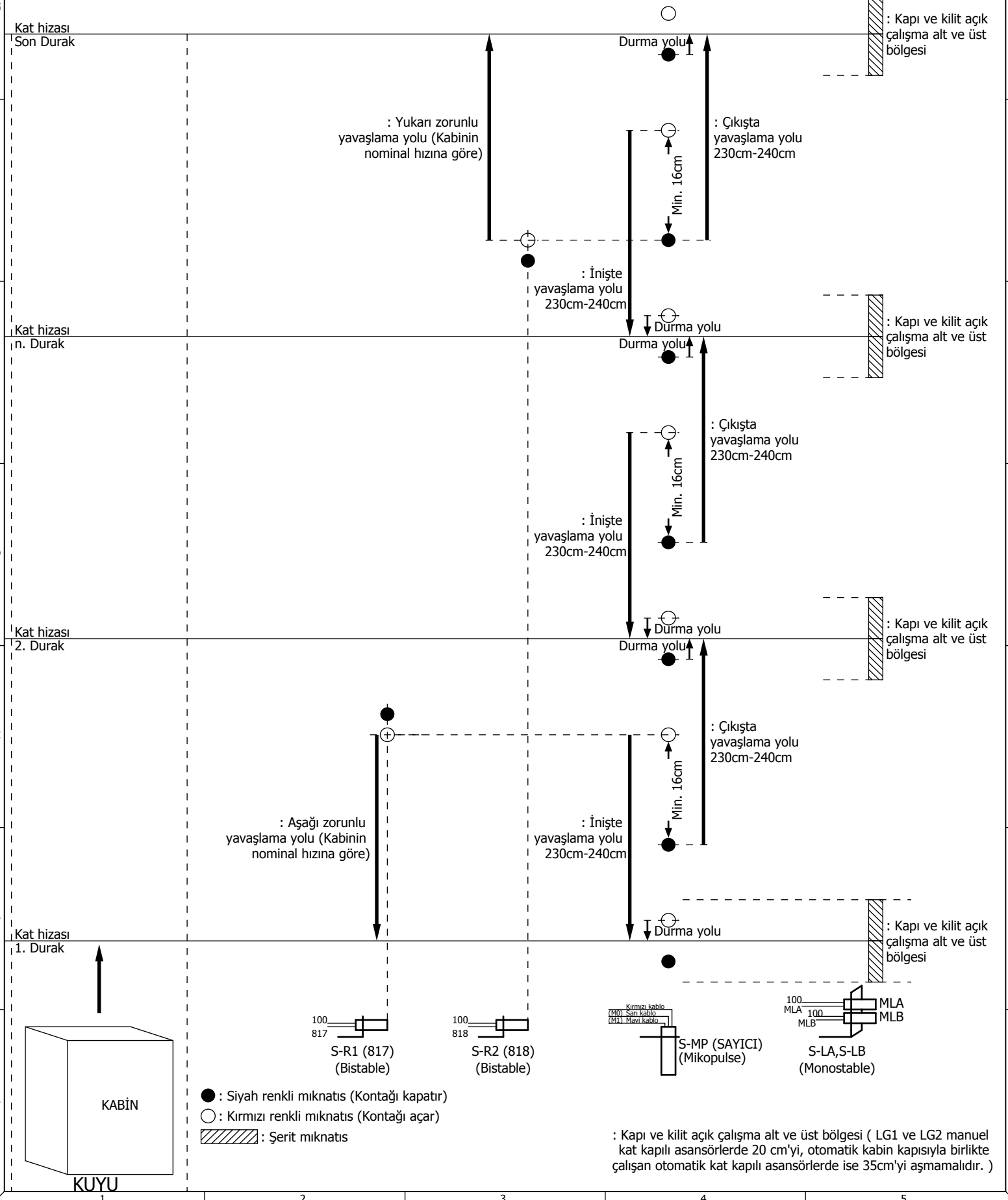
MIKNATIS DİZİLİM ŞEMASI PAKET 2 (SAYICI + SEVİYE DÜZELTME) "1. mıknatıs değişik"
