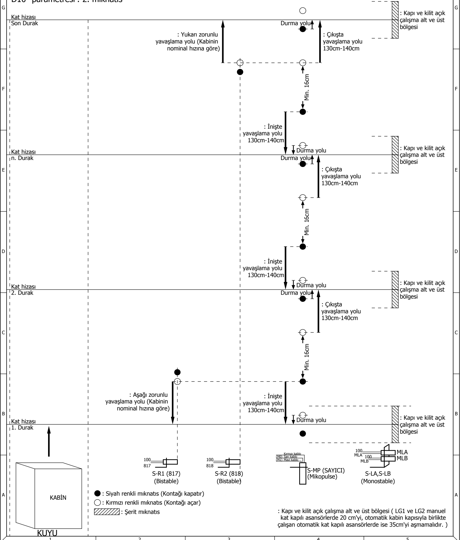
MIKNATIS DİZİLİM ŞEMASI PAKET 2 (SAYICI + SEVİYE DÜZELTME) "2. mıknatıs değişik"
