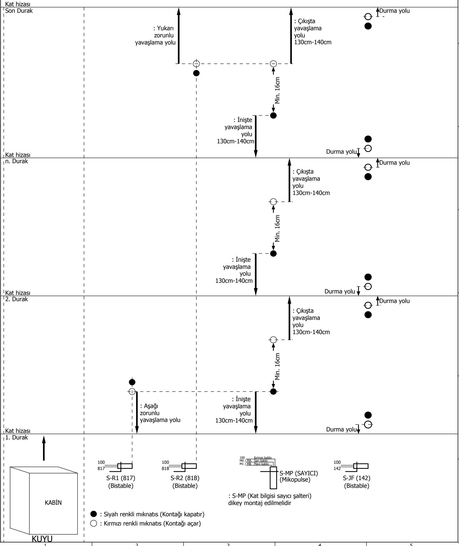
MIKNATIS DİZİLİM ŞEMASI PAKET 3 (SAYICI + 142 JF) "2. mıknatıs değişik"
