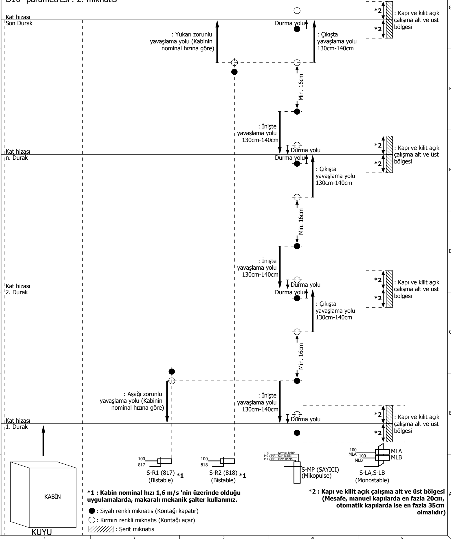
MİKNATIS DİZİLİM ŞEMASI PAKET 2 (SAYICI + SEVİYE DÜZELTME) "2. mıknatıs değişik"
