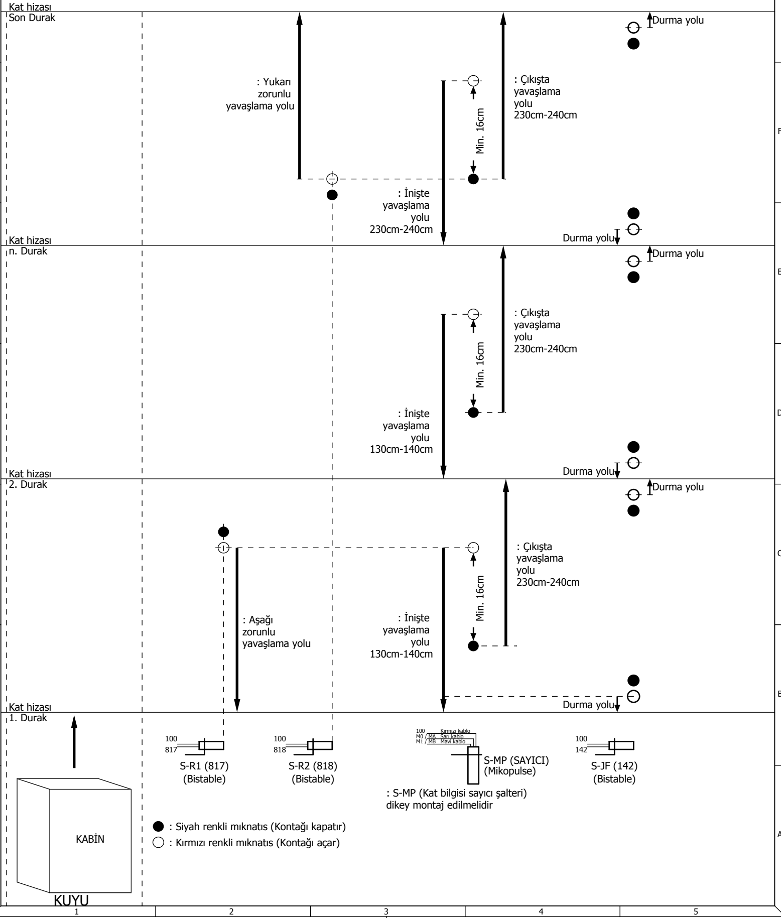
MIKNATIS DİZİLİM ŞEMASI PAKET 3 (SAYICI + 142 JF) "1. mıknaş değişik"
