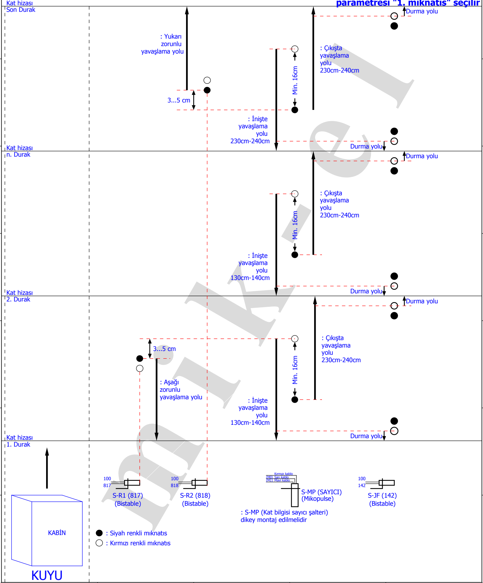
MIKNATIS DİZİLİM ŞEMASI PAKET 3 (SAYICI + JF(142)) "1. mknatis deęiş"
